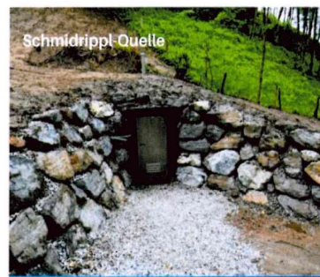
„Quellstube“ Schmidrippel-Quelle
