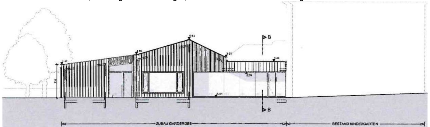
ANSICHT NORD 1:100
